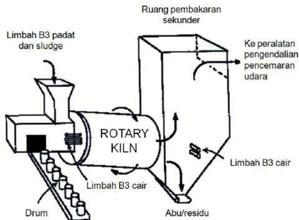
Gambar 3. Contoh insinerator tipe statis dan tipe rotari.
