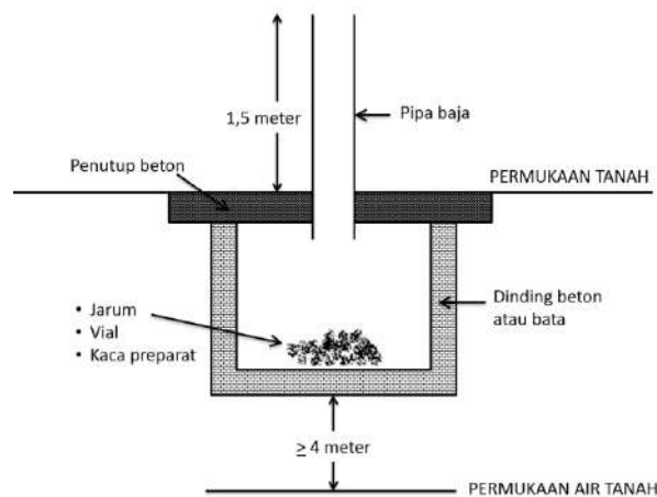
Gambar 1. Sketsa fasilitas penguburan limbah benda tajam.
